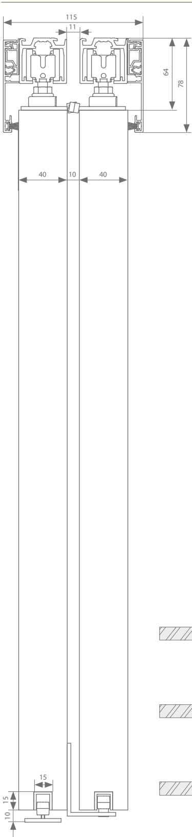
Parallelle plafondbevestiging 2
