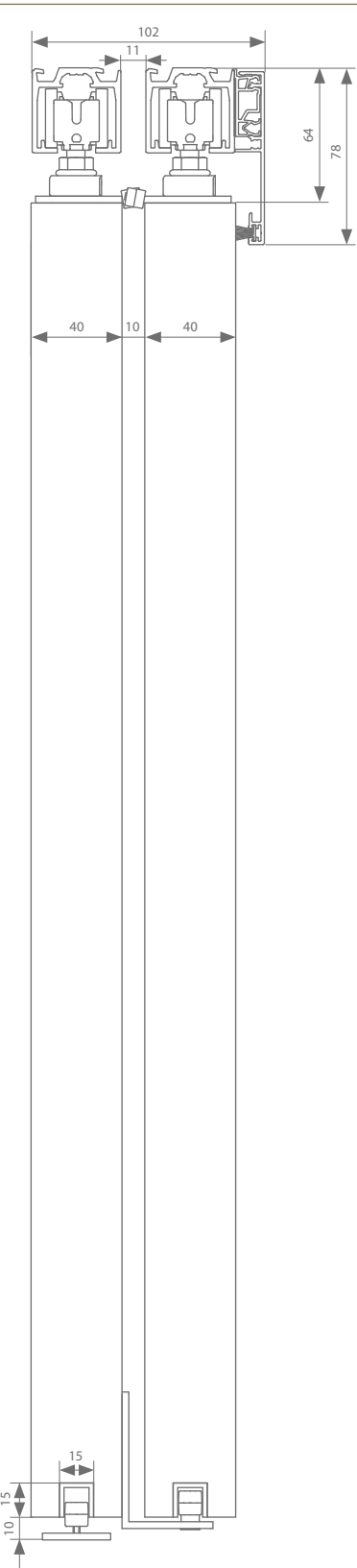
Parallelle plafondbevestiging 1
