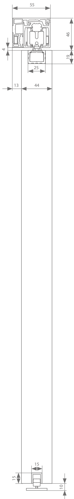
Muurbevestiging 44 mm
