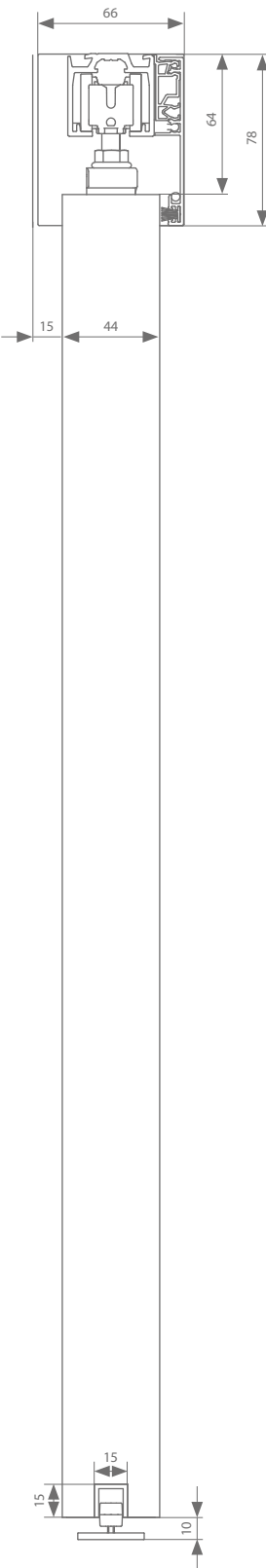
Plafondbevestiging 44 mm
