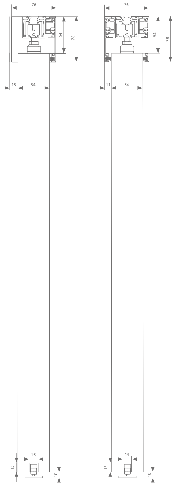
Plafondbevestiging 54 mm
