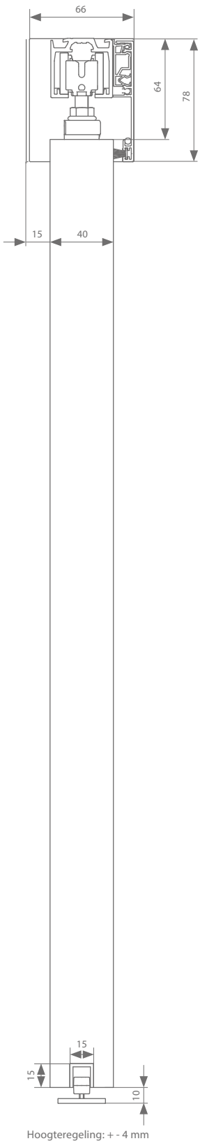
Plafondbevestiging 40 mm
